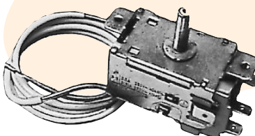
SELNEV TB.08A808 ATEA A13.0068
