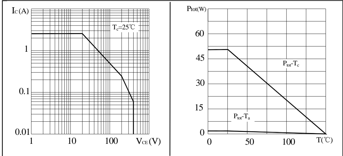
图2 P_{tot}-T 关系曲线
