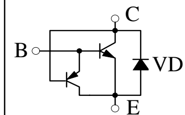
内部等效原理图
