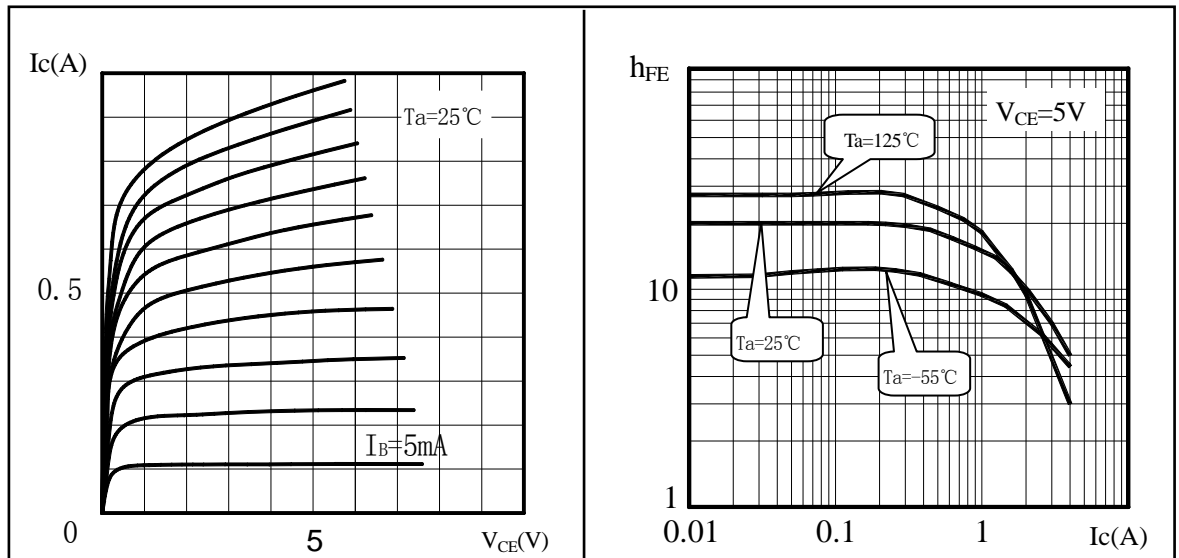
图3 输出特性曲线 ( I_C-V_{CE} )
