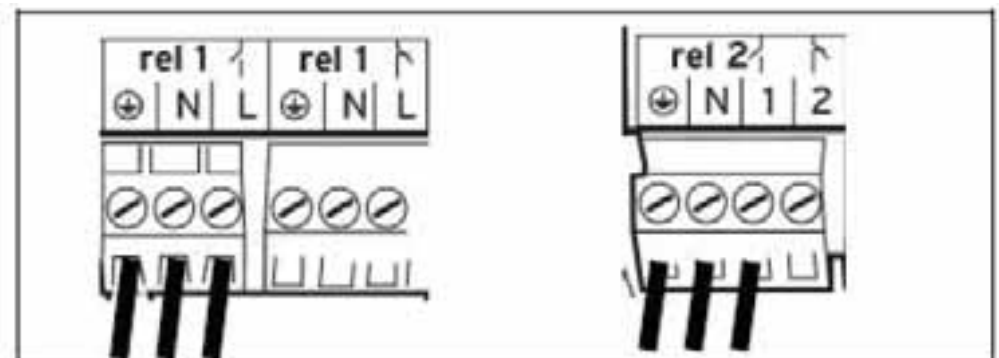
Подключение внешнего насоса нагрева водонагревателя
