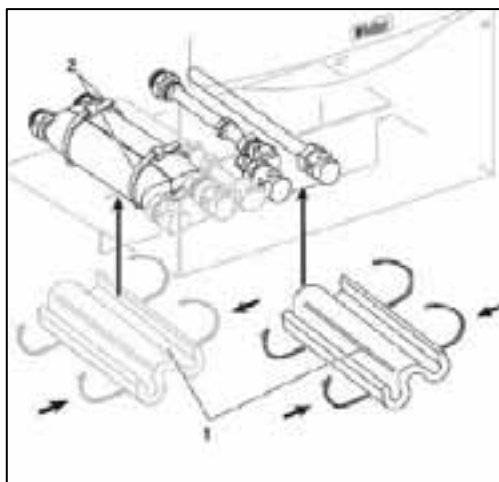
Рис. 5.4 Установка теплоизоляции
