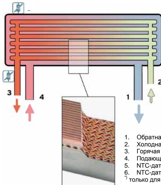
Вторичный теплообменник с NTC-датчиком (котлы серии plus)
