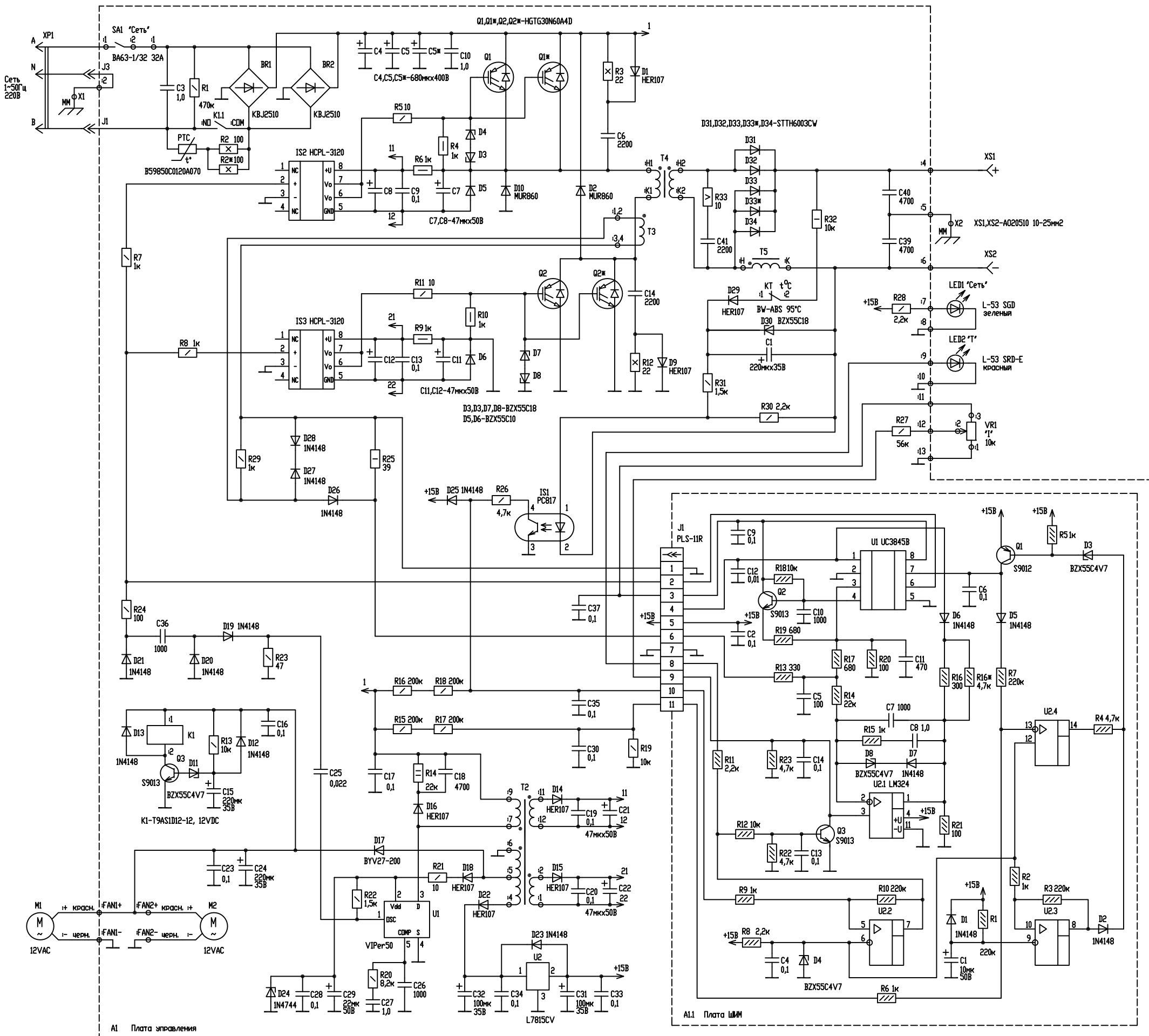
Схема электрическая принципиальная выпрямителя ВД-200 "Ресанта"
