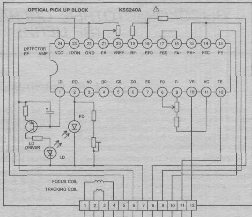
Рис. 3.4. Оптический преобразователь KSS240A в состав которого входит RF усилитель
