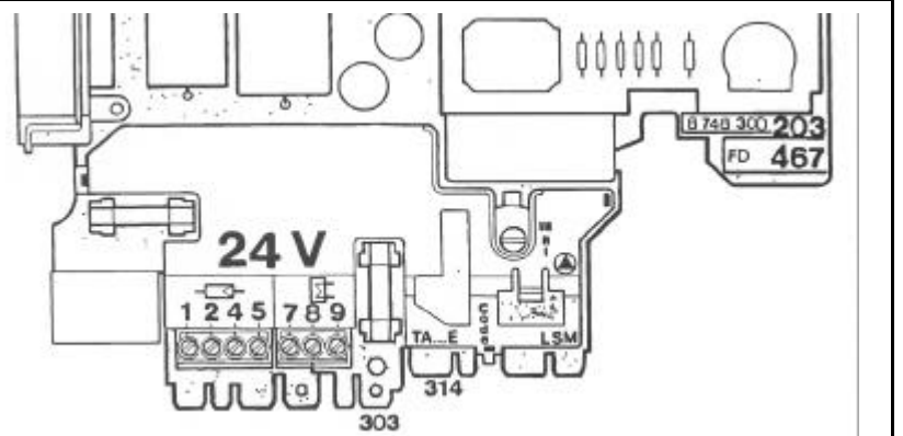
Fig. 10 303 klemmen voor NTC boiler 314 klemmen voor inbouwregelaar TA 210 E (24 V/DC) 303 bornes pour CTN boiler 314 bornes pour régulateur à ncorprer TA 210 E (24 V/DC)
