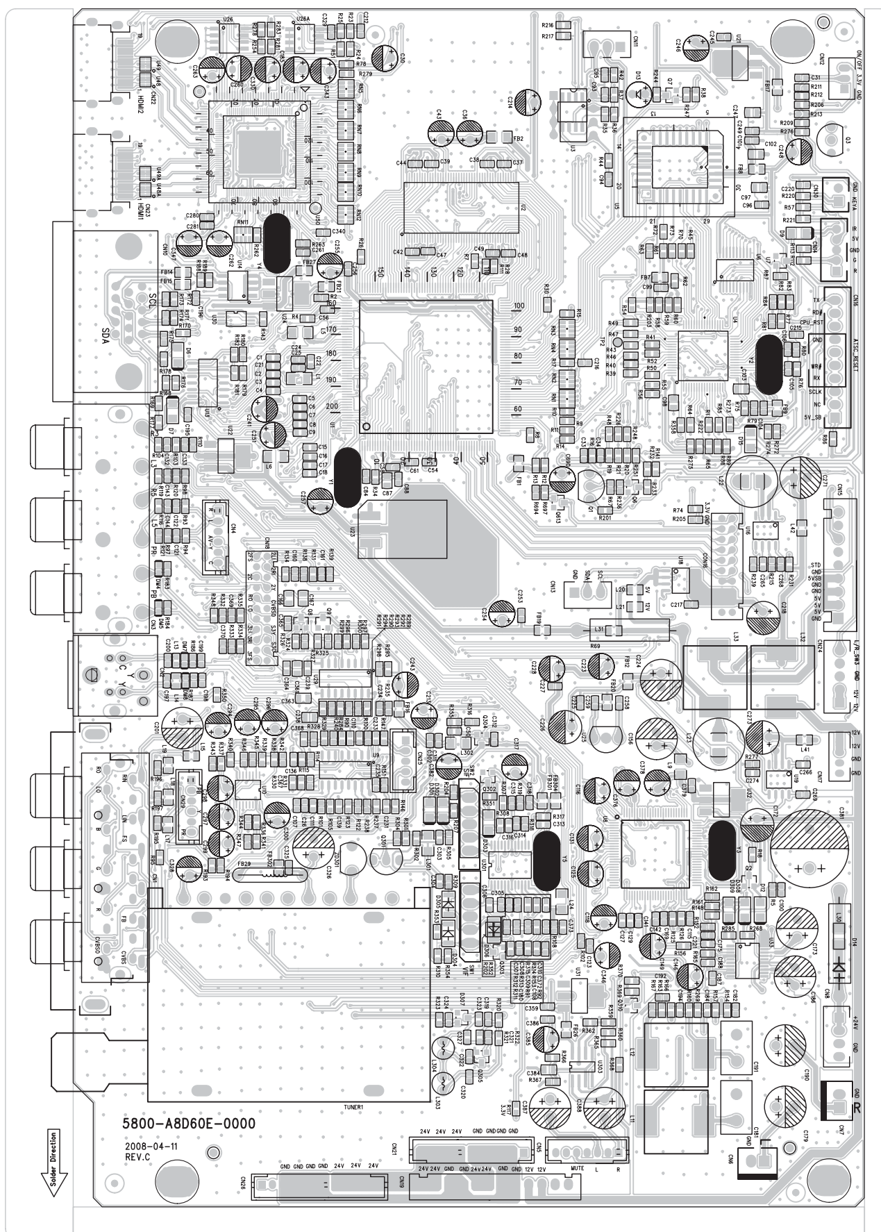
Main PCB top layer
