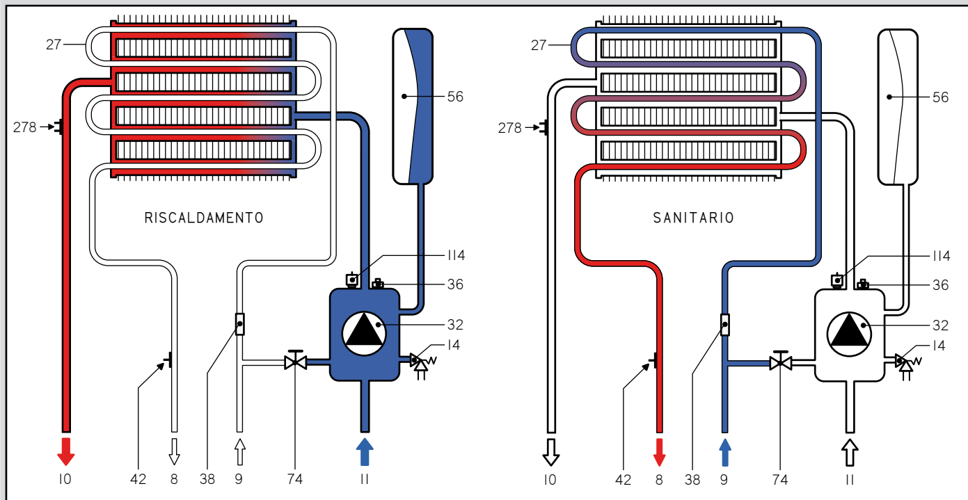
schema idraulico attualmente in produzione
