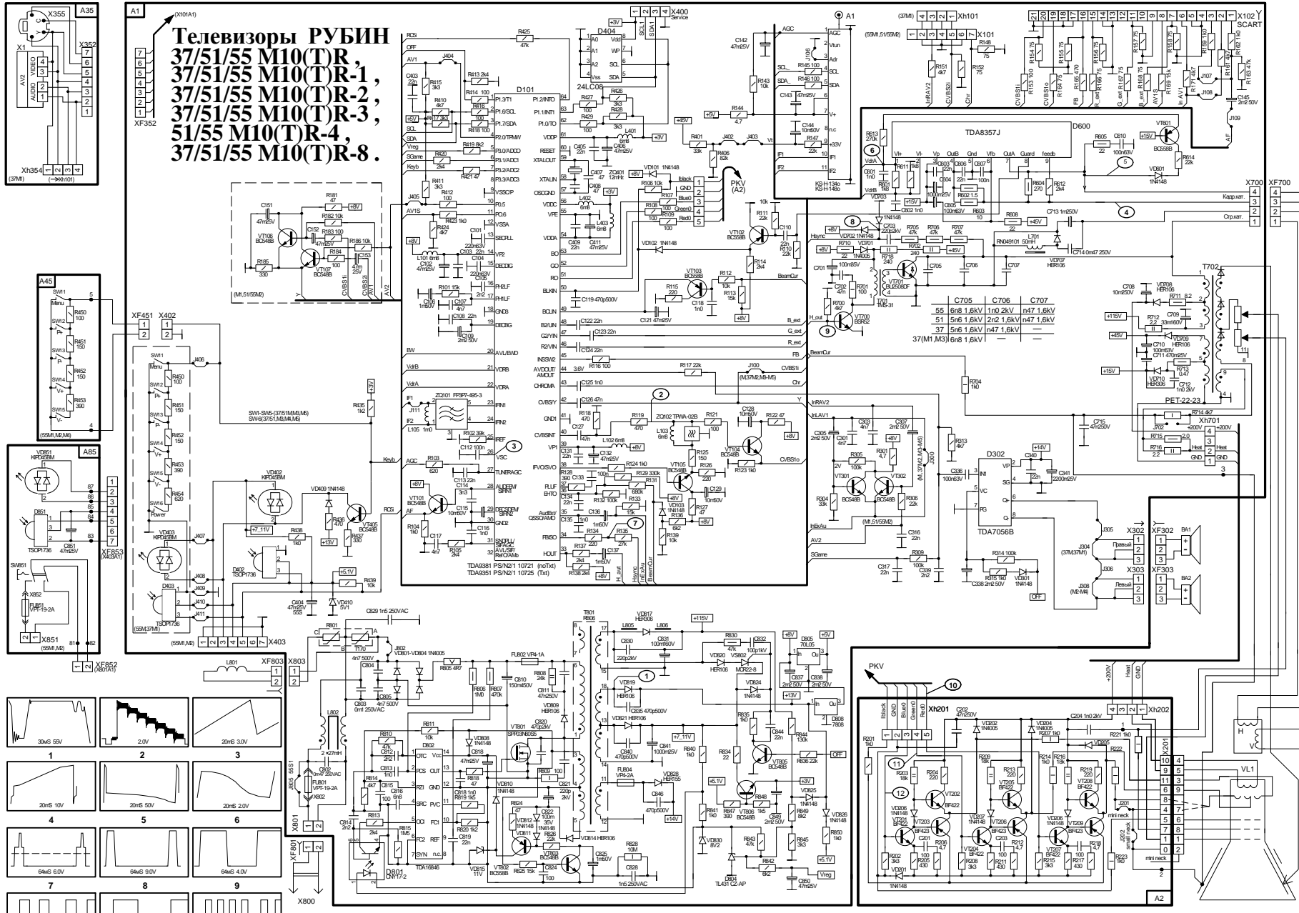
Осциллограммы в контрольных точках приведены при приеме сигнала "Летний полос". Показан период и размах.
