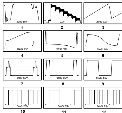
Осциллограммы в контрольных точках приведены при приеме сигнала "Летний полос". Показан период и размах.
