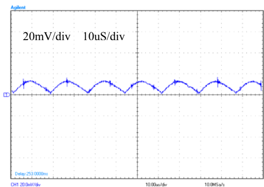
Vin=85V, Io=1A
