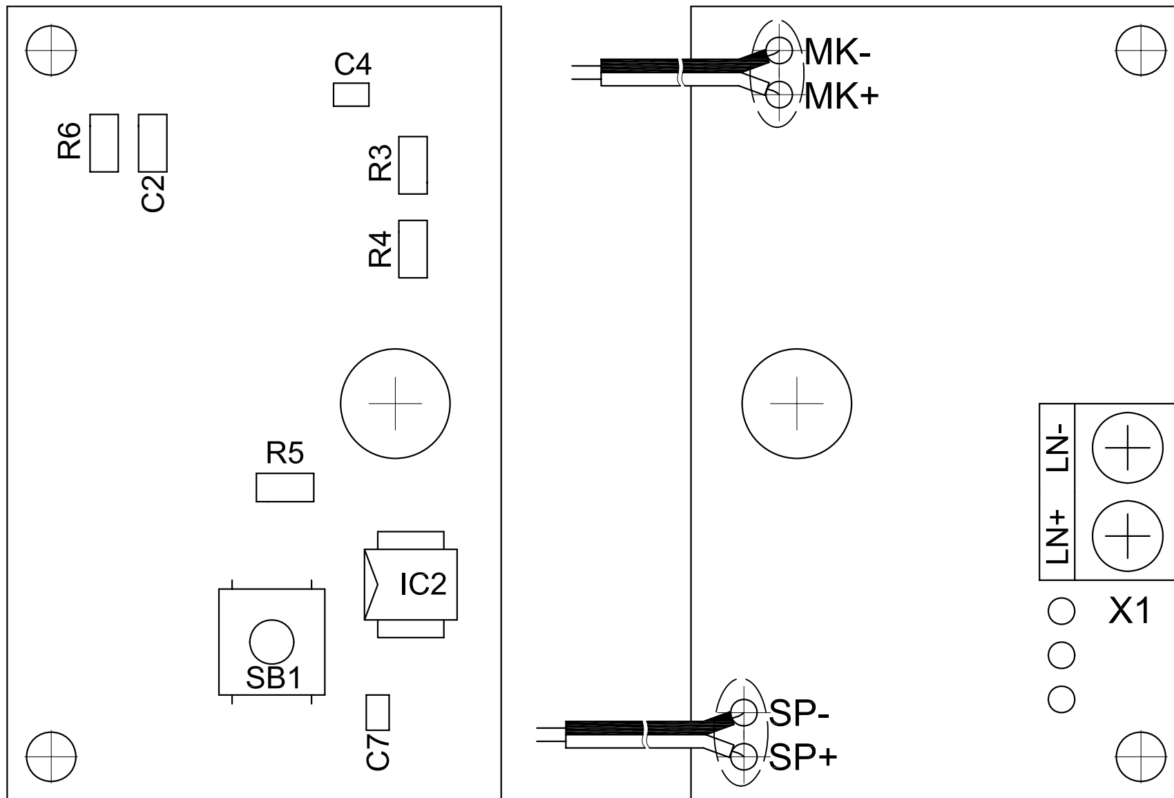
Плата БВД-104А Сборочный чертеж
