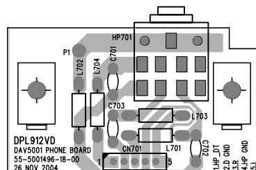
Headphone-jack P.C.B. Platine prise-casque Ltpl. Kopfhörerbuschse Piastra presa per cuffia Platina toma auriculares
