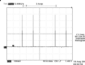
2 U501-#44 V-SYNC
