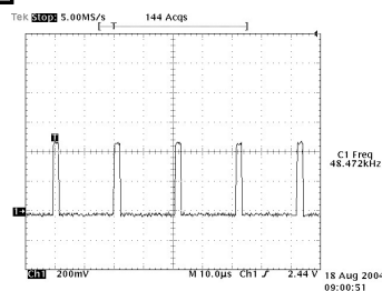
2 U501-#43 H-SYNC
