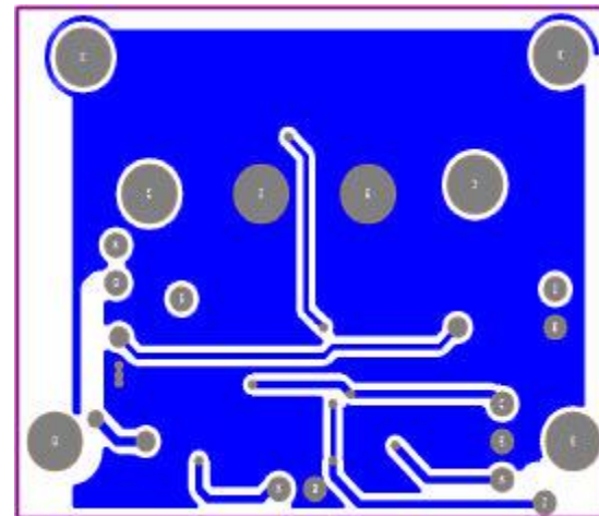
Bottom Layer
