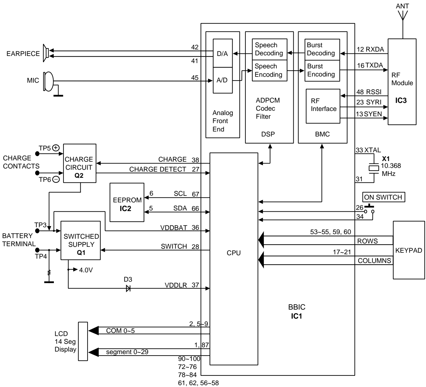
KX-A141RUM/RUS&142RUM/RUS BLOCK DIAGRAM (HANDSET)
