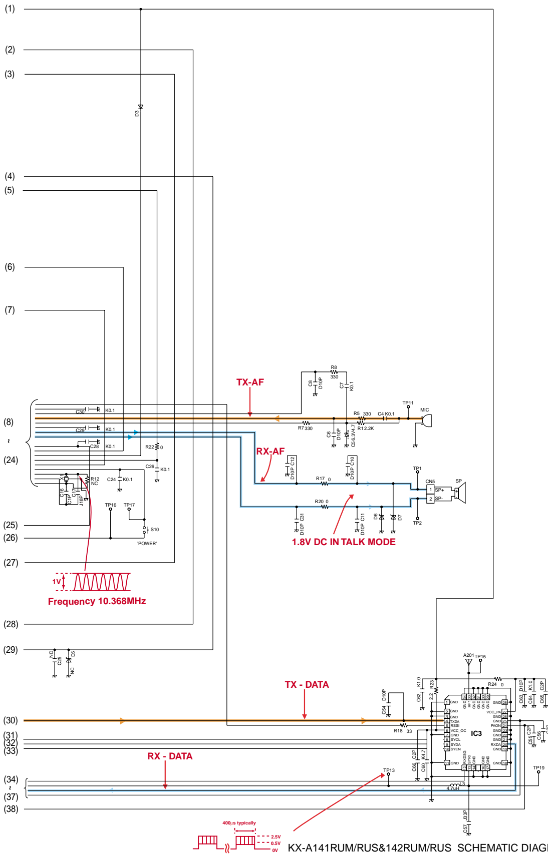
KX-A141RUM/RUS&142RUM/RUS SCHEMATIC DIAGRAM (HANDSET)
