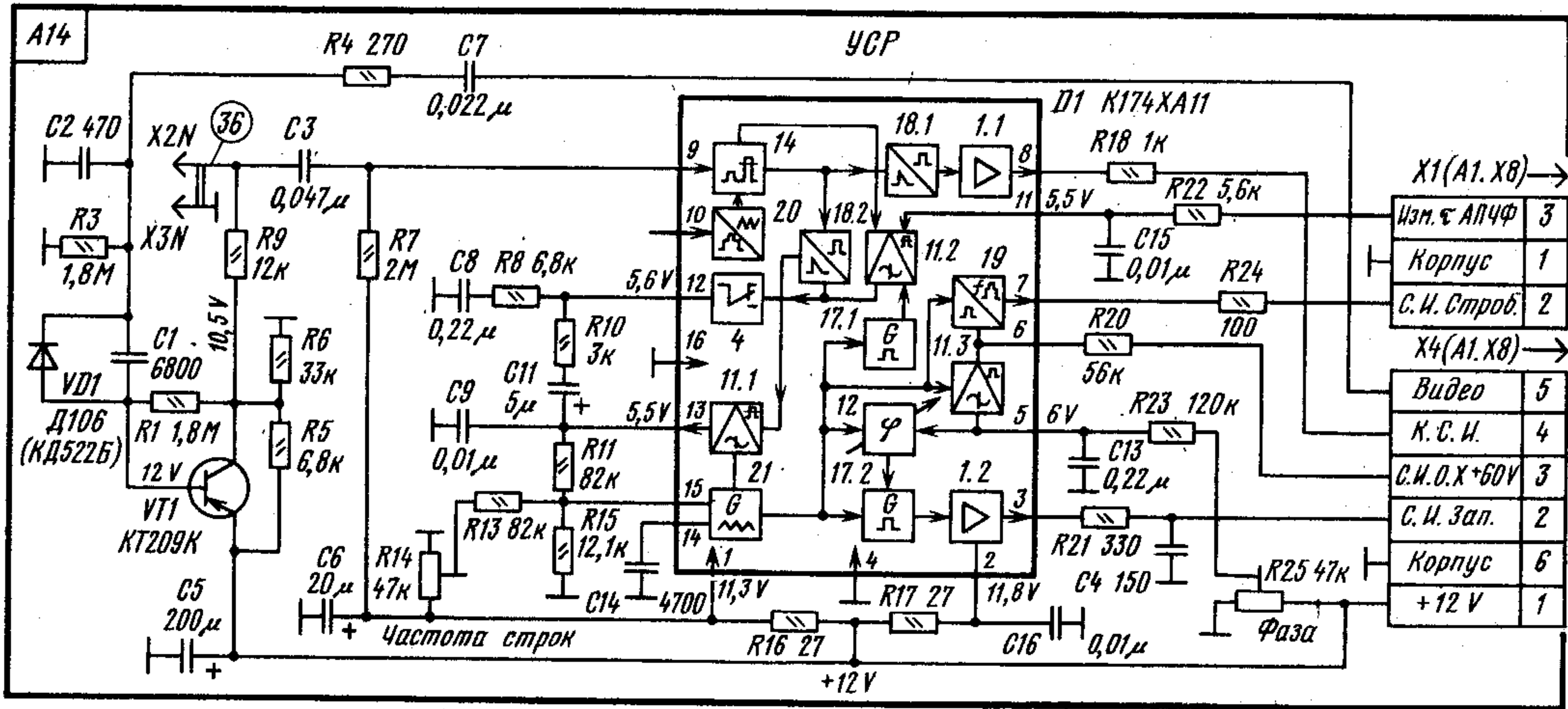
Принципиальная схема submodule синхронизации УСР
