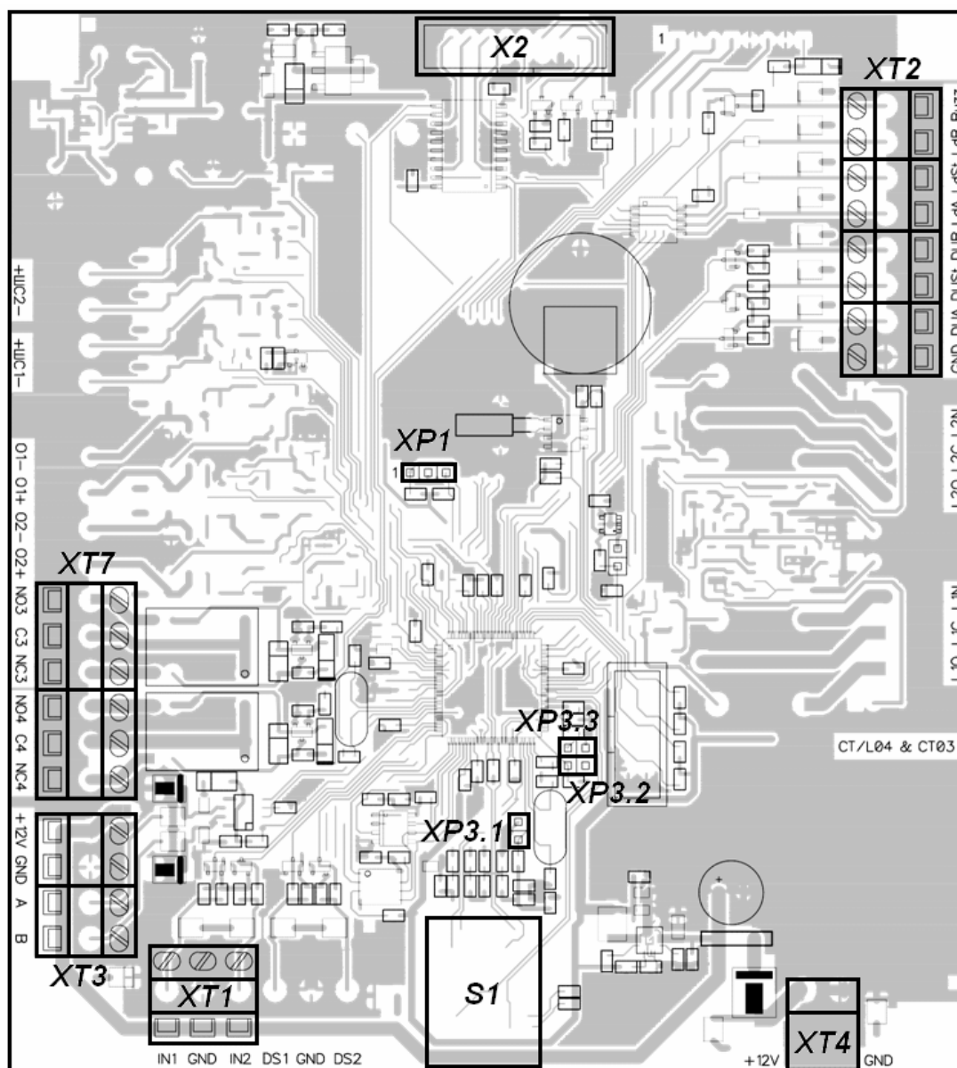
Рисунок 3 Плата контроллера PERCo-CT03
