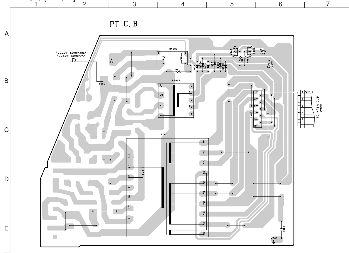
WIRING-3 [PT C.B.]
