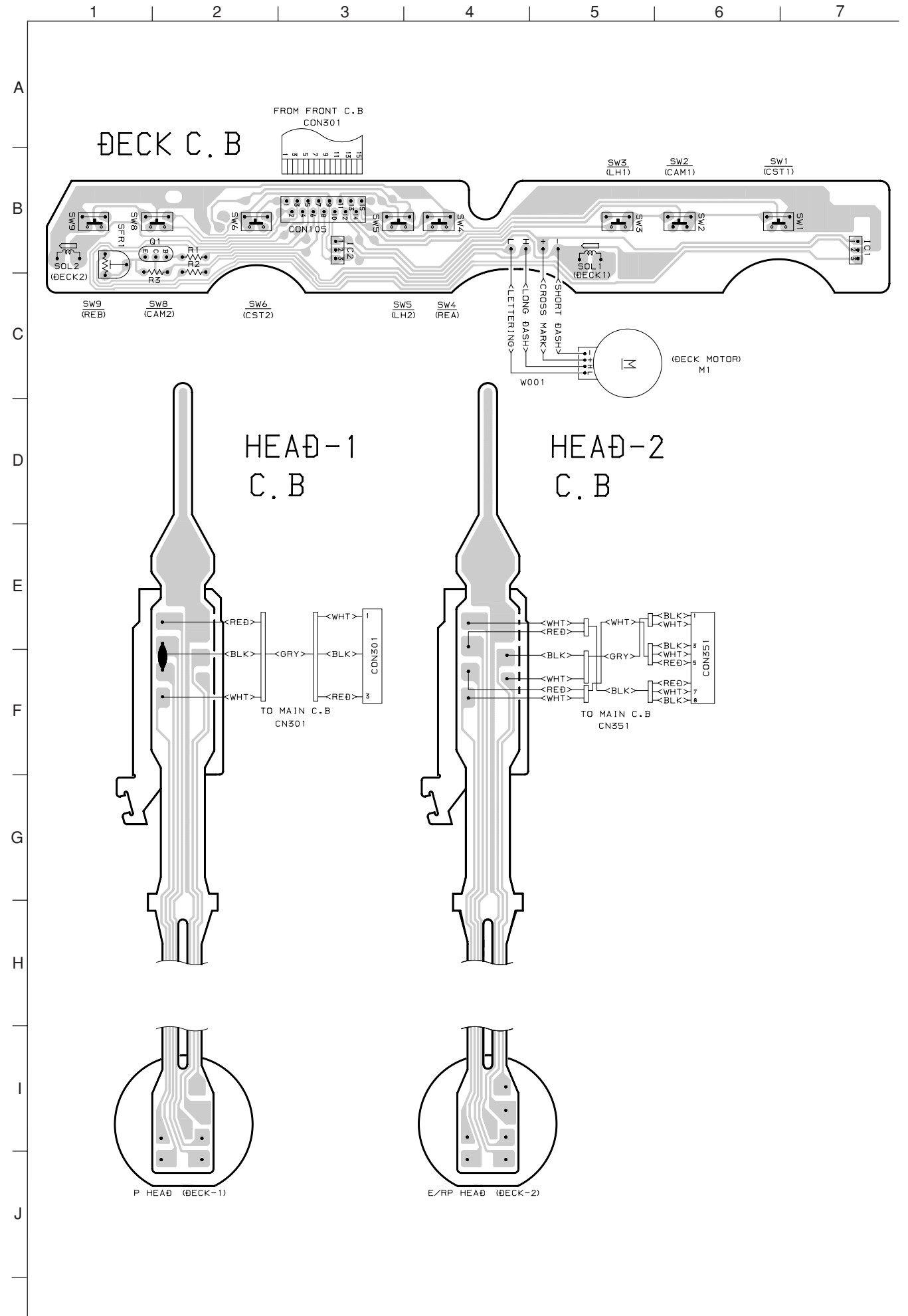
WIRING-4 [DECK C.B.] <HS>
