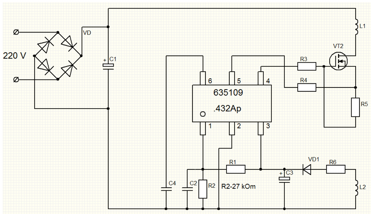
Фрагмент схемы на микросхеме с кодовым названием .432Ap
