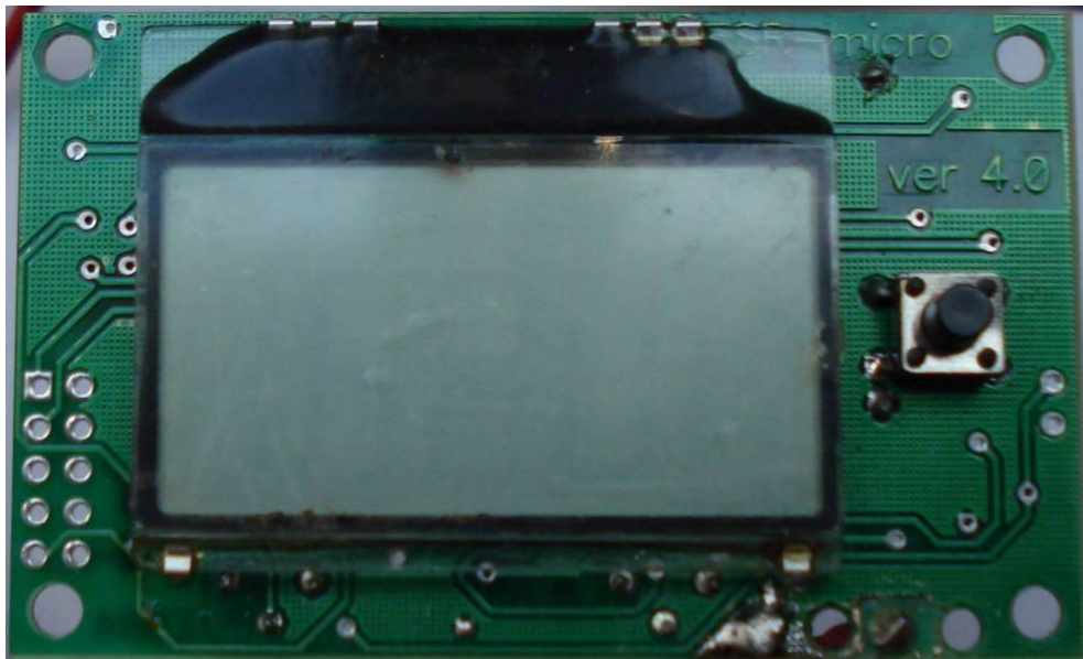
Рис.2 Плата спереди
