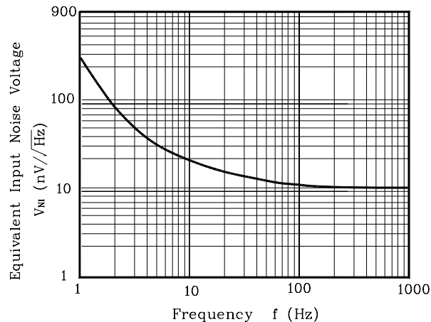
Fig. 6 V_{NI} - f
