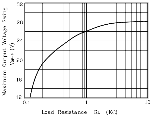
Fig. 5 V_{OP-P} - R_L
