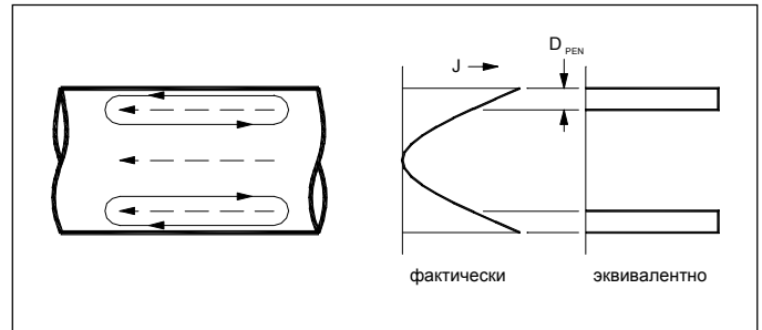
Рис.3 Распределение тока на высокой частоте
