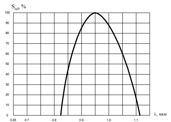
Рисунок 2 – Зависимость чувствительности от длины волны ИК-излучения при T_{amb} = 25^\circ\text{C} (спектральная характеристика).
