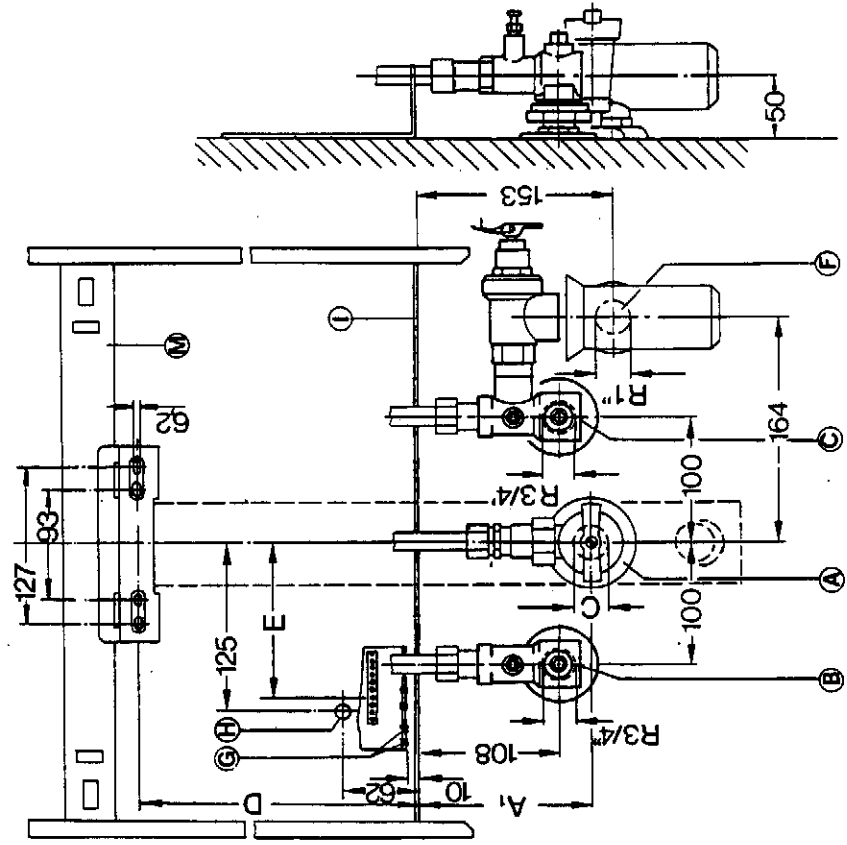
Соединительные размеры скрытый монтаж
