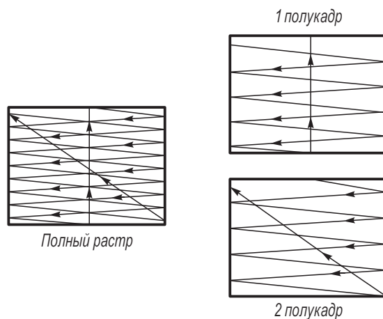
Рис. 1.11. Ход лучей кинескопа при чересстрочной развертке
