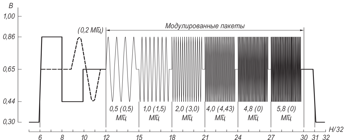
Рис. 1.29. Комбинированный сигнал 1
