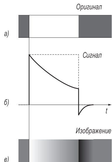
Рис. 1.14. Искажения типа «тянущиеся продолжения»
