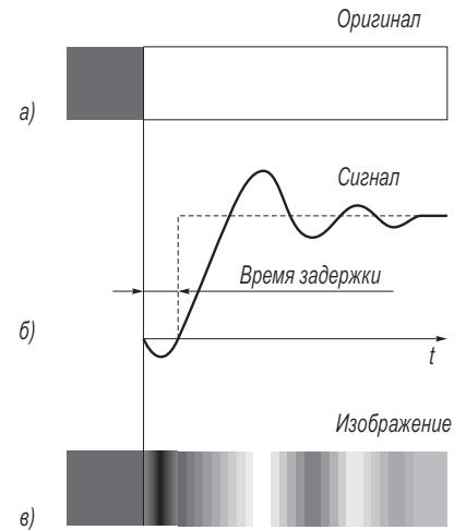
Рис. 1.17. Искажения типа «оконтуривание»
