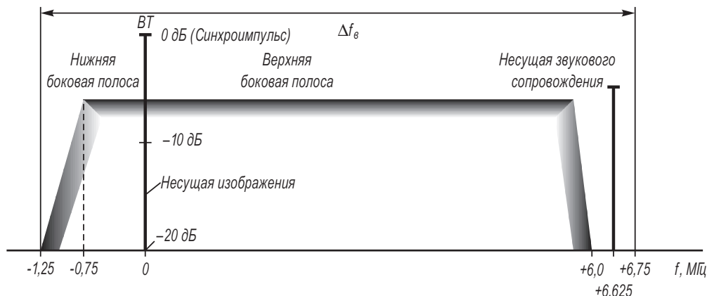
Рис. 1.3. Спектр полного телевизионного сигнала
