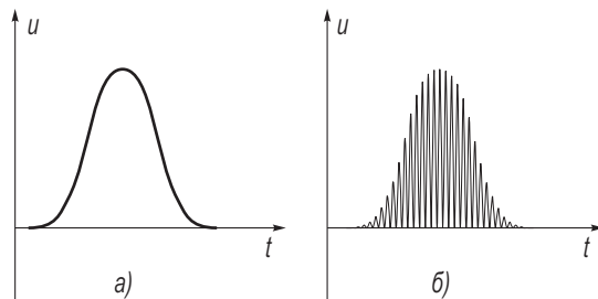
Рис. 1.25. Синусквадратичные импульсы
