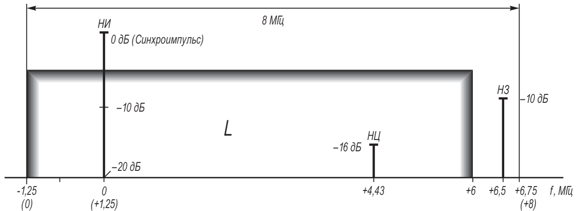
Рис. 1.7. Спектр телевизионного стандарта L
