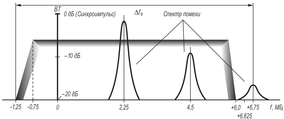
Рис. 1.36. Спектр сигнала при наложении сигнала помехи
