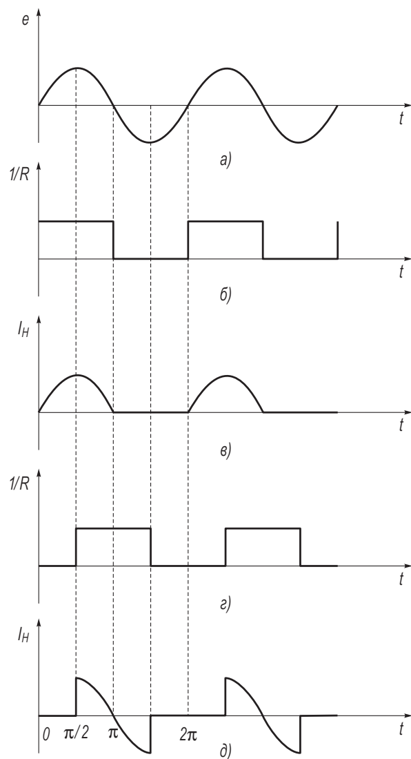
Рис. 1.19. Синхронный детектор, эюры сигналов
