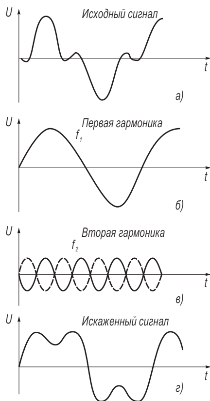
Рис. 1.20. Спектральный состав прямоугольного сигнала
