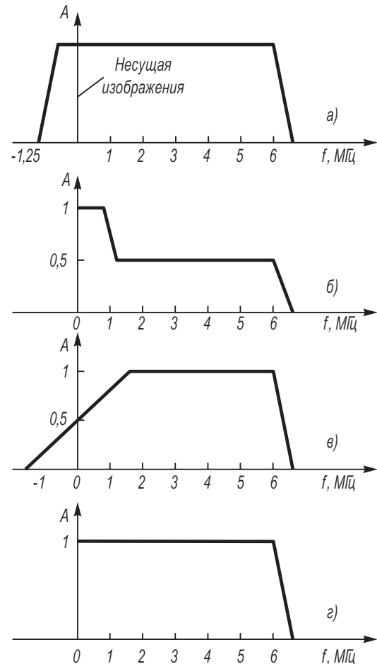
Рис. 1.10. Формирование АЧХ видеодетектора
