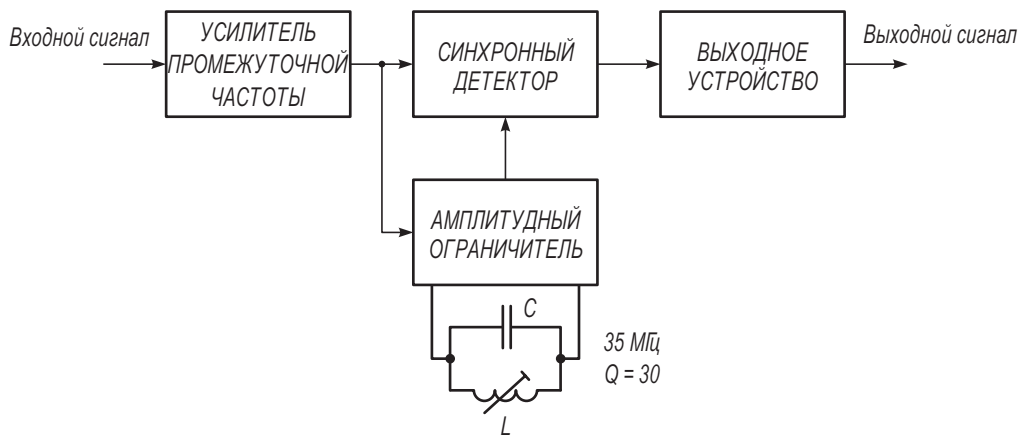
Рис. 1.18. Структурная схема синхронного детектора
