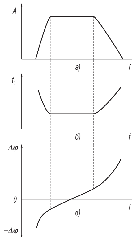
Рис. 1.21. Связь амплитудно-частотной и фазо-частотной характеристик сложного сигнала
