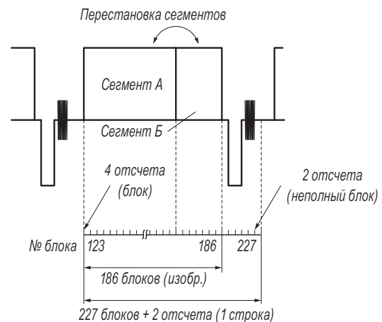
Рис. 1.34. Коммутация видеосигнала в пределах строки
