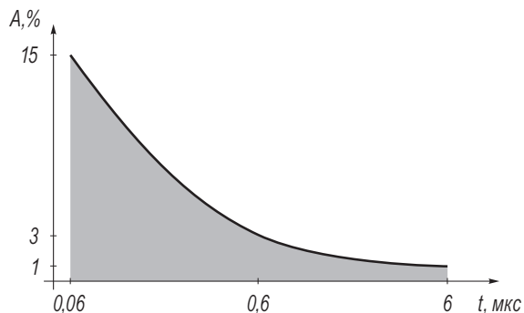
Рис. 1.16. Зависимость искажений цвета от интенсивности мешающего сигнала
