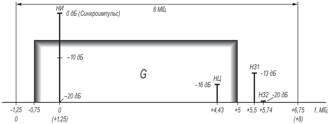
Рис. 1.4. Спектр телевизионного стандарта G
