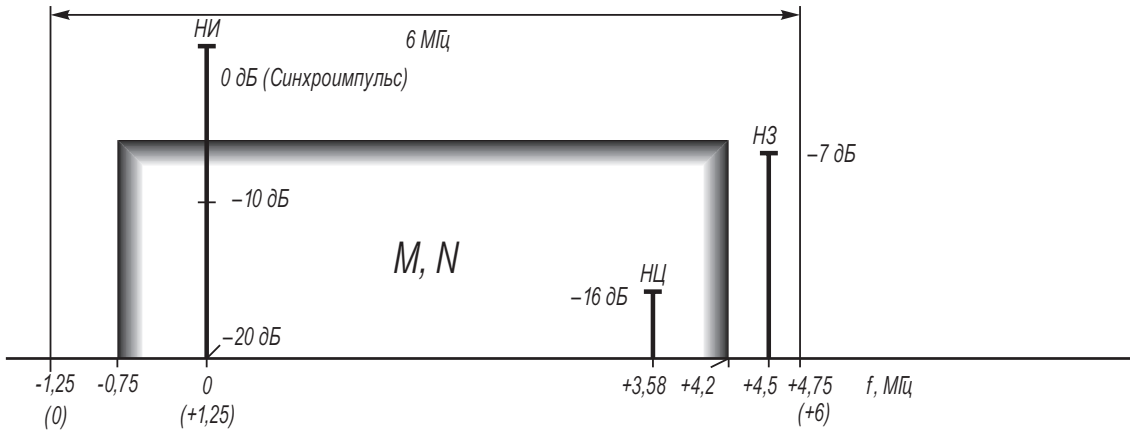
Рис. 1.5. Спектр телевизионных стандартов M, N
