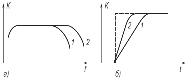
Рис. 1.15. Изменение полосы пропускания тракта изображения
