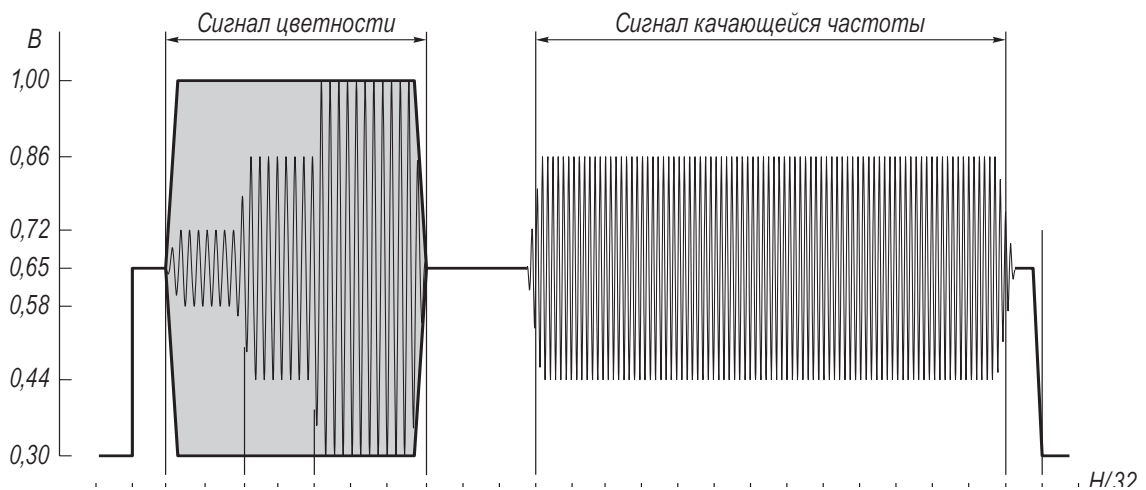
Рис. 1.32. Комбинированный сигнал 4
