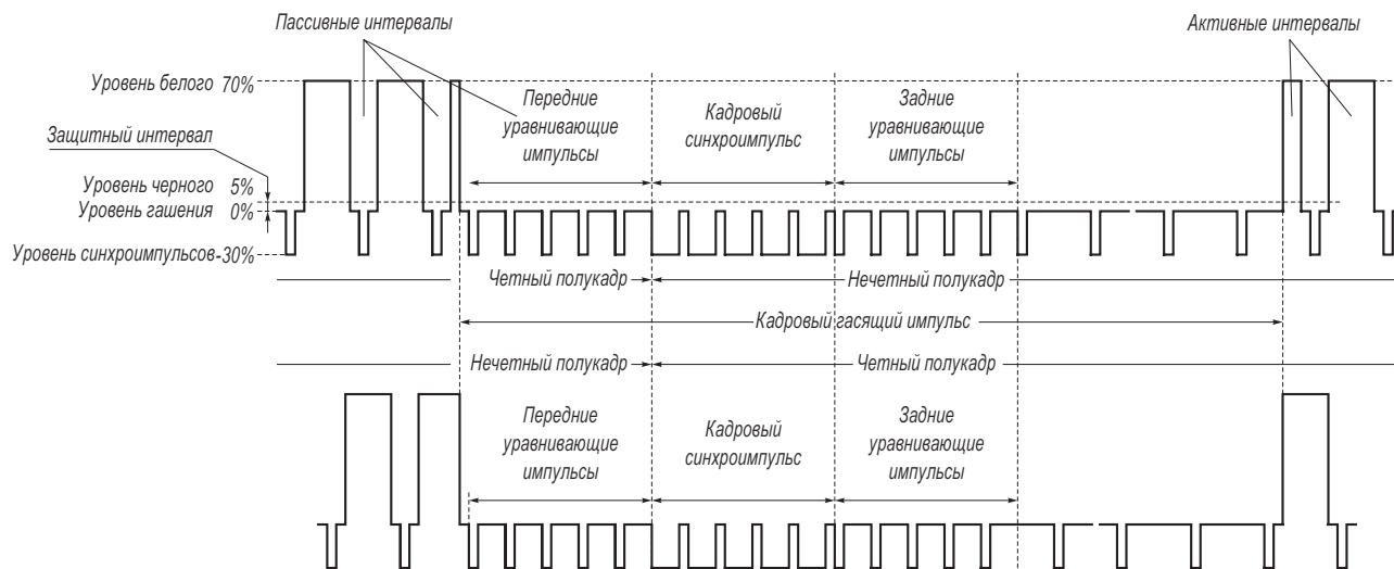
Рис. 1.2. Полный видеосигнал
