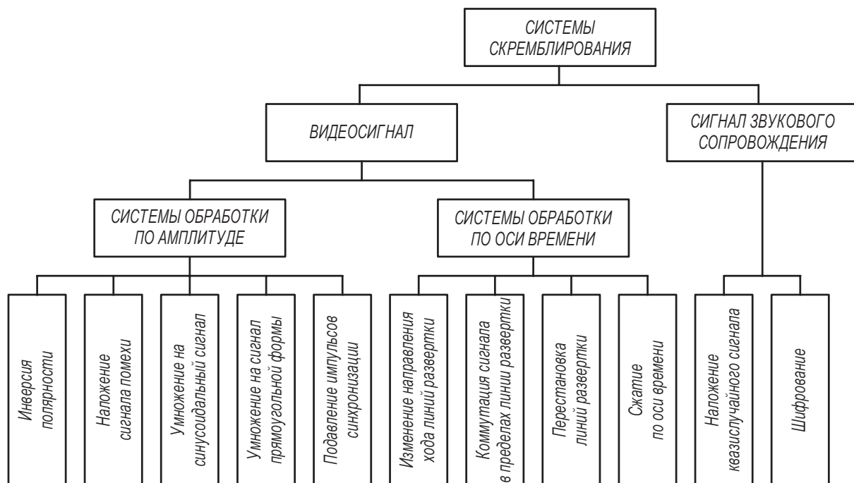
Рис. 1.33. Методы скремблирования сигналов
