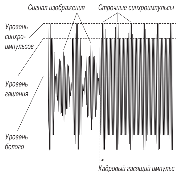
Рис. 1.8. Телевизионный радиосигнал
