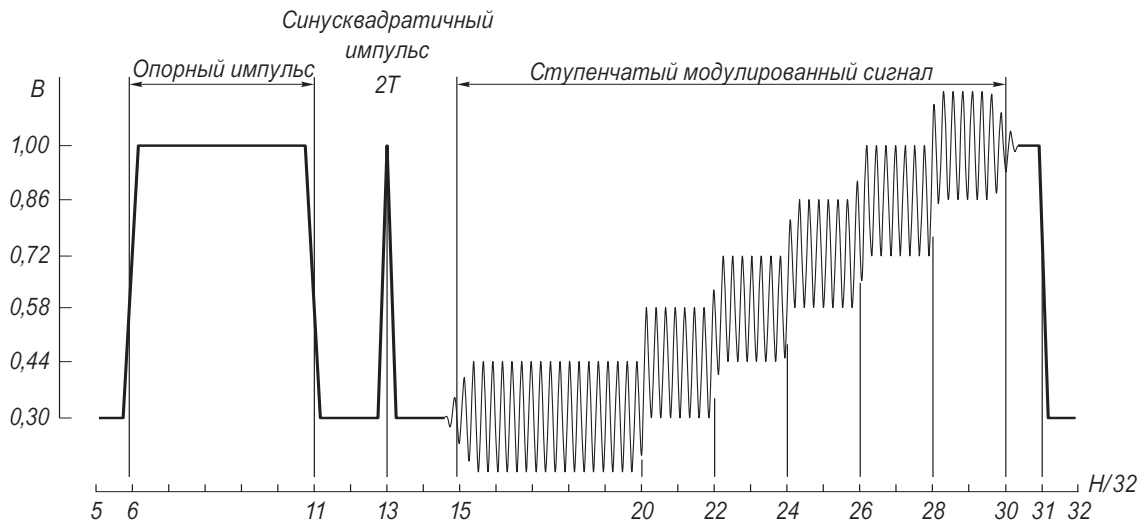
Рис. 1.31. Комбинированный сигнал 3
