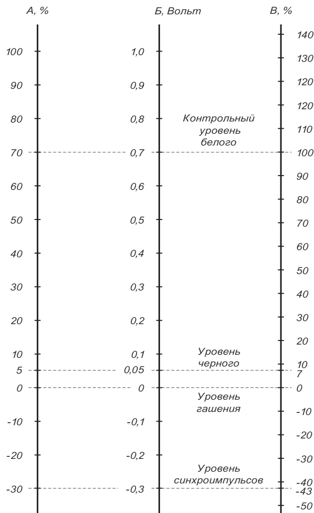
Рис. 1.12. Шкалы для контроля уровней видеосигналов
