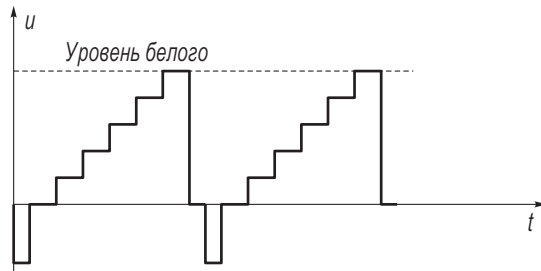
Рис. 1.22. Сигнал ступенчатой формы
