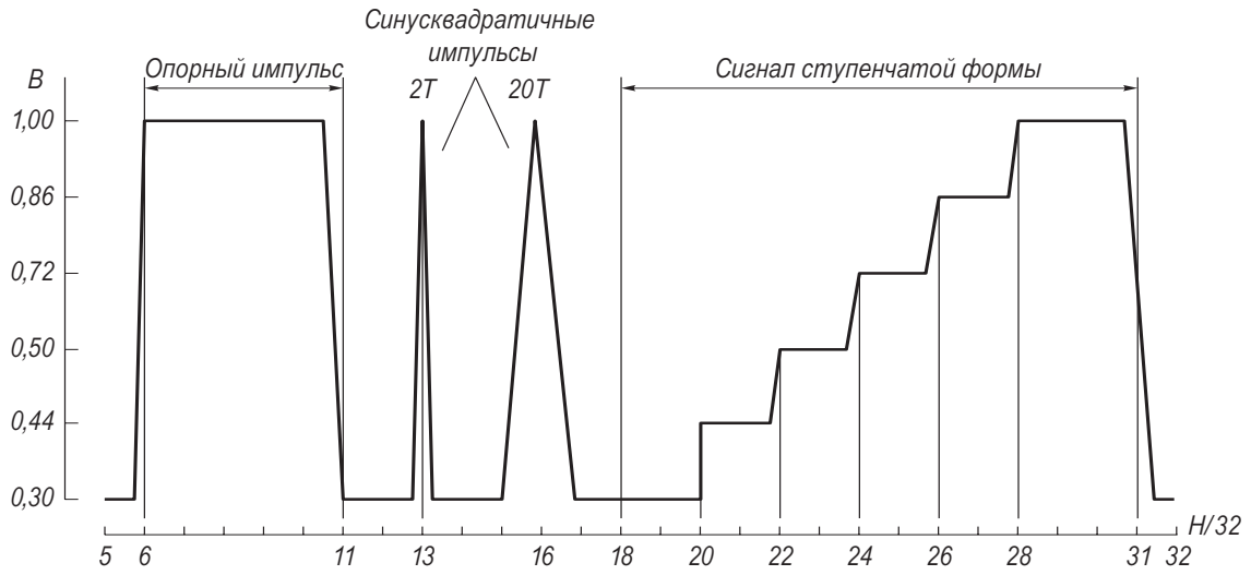
Рис. 1.30. Комбинированный сигнал 2
