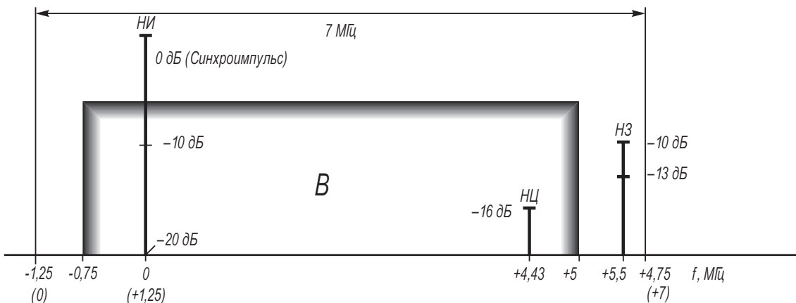
Рис. 1.6. Спектр телевизионного стандарта B
