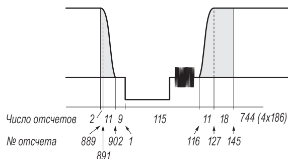
Рис. 1.35. Дополнительные отсчеты в скремблированном сигнале
