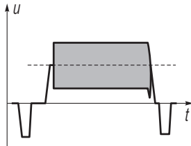
Рис. 1.28. Искажения огибающей частотно-модулированного сигнала
