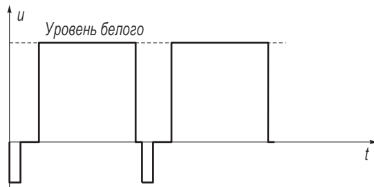
Рис. 1.24. Сигнал прямоугольной формы
