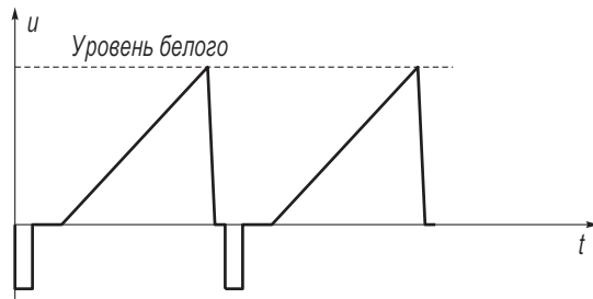
Рис. 1.23. Сигнал пилообразной формы
