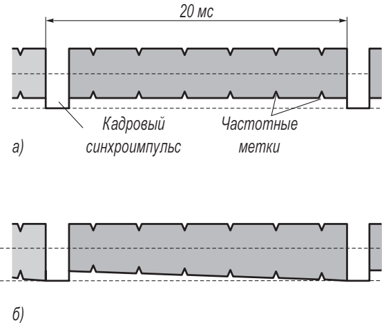
Рис. 1.27. Сигналы качающейся частоты
