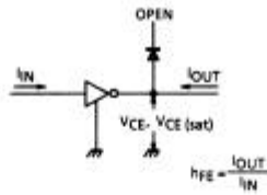
2. V_{CE(sat)} , h_{FE}
