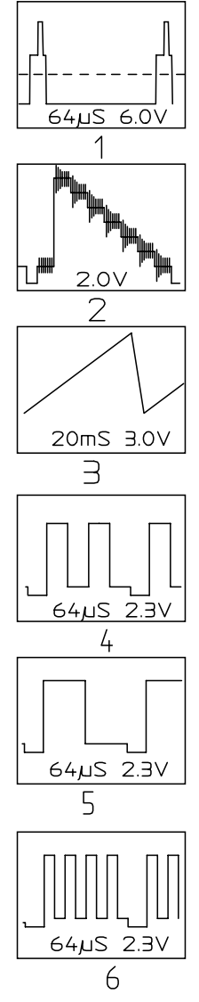
Осциллограммы в контрольных точках приведены при приеме сигнала "Цветные полосы". Указан период и размах.
