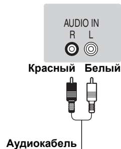
Тыльная панель усилителя
