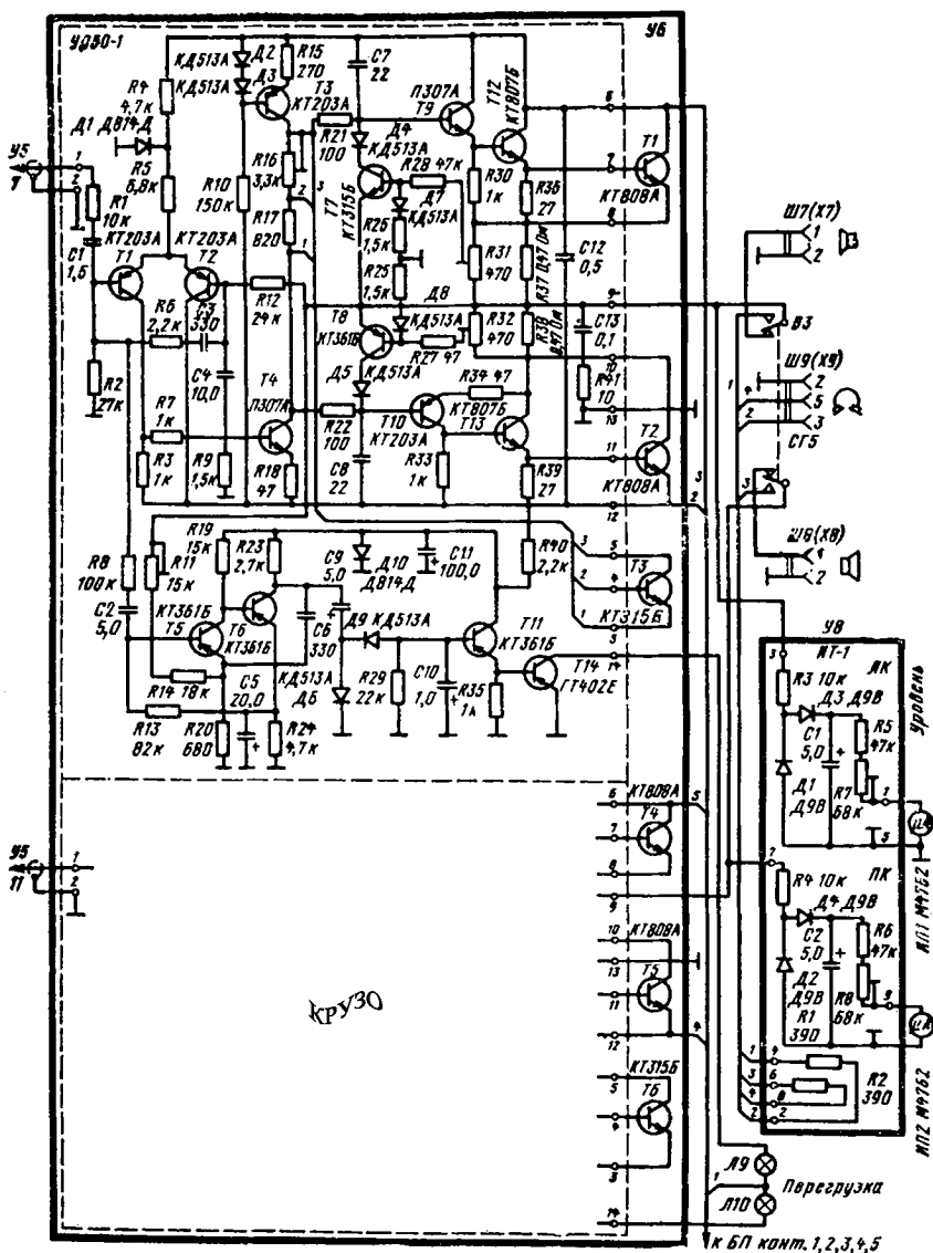
Принципиальные электрические схемы оконечного усилителя с электронной защитой УО50-1 (У6) и выпрямителя выходного сигнала для индикатора ИТ-1 (У8) электрофона «Аллегро-002-стерео» и УКУ «Радиотехника-020-стерео»
