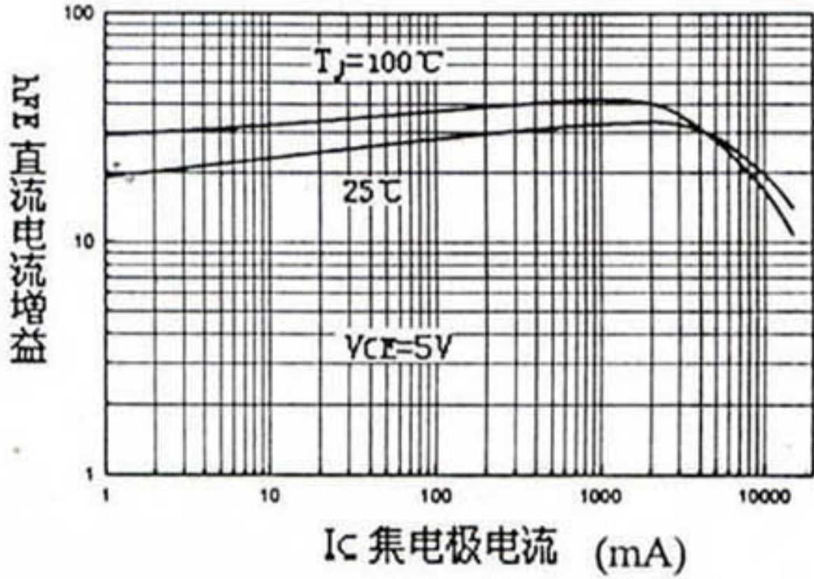
百流增益-集电极电流特性
