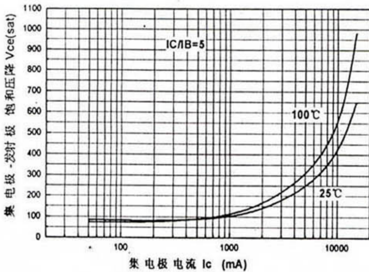
饱和压降-集电极电流特性
