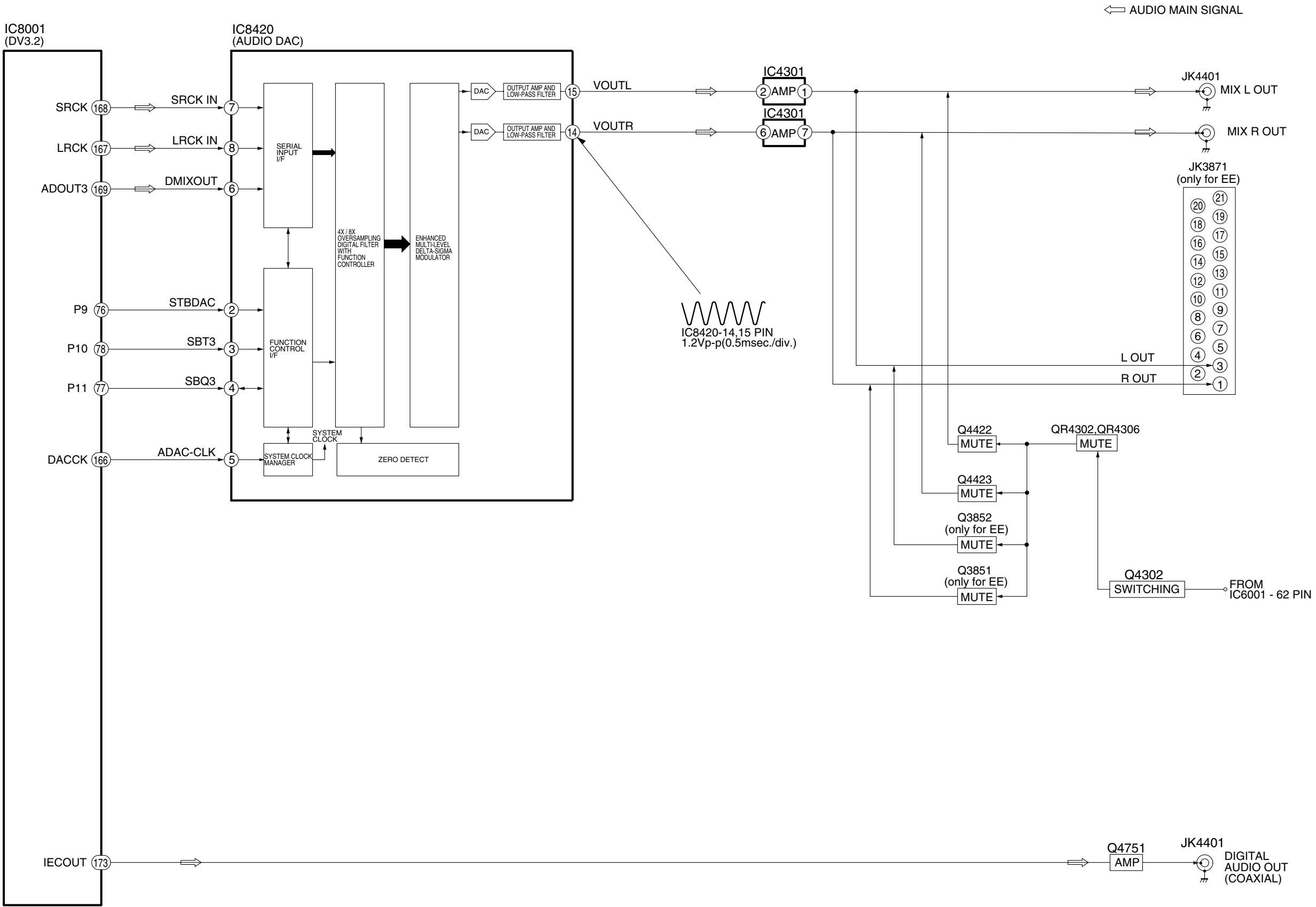
DVD-S42EE/GC/GCA/GCS/GCU/PL/PLA AUDIO BLOCK DIAGRAM
