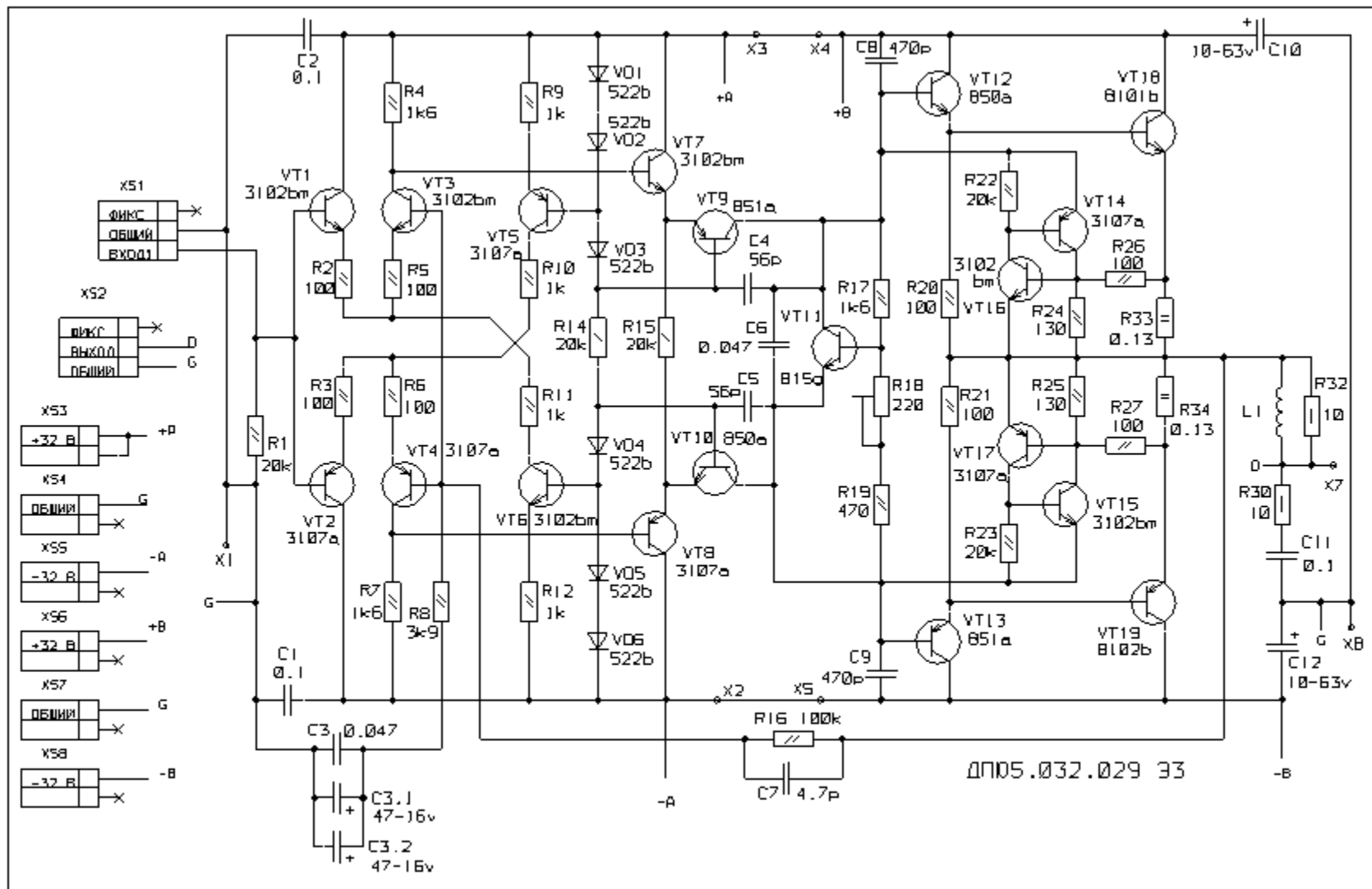
Узел усилителя мощности 50 W \ 4 Ом ( А4546 УМ0545 УМ0547 )
