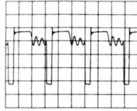
⑰ 440 Vp-p (H)
