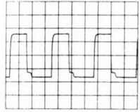
⑥ 3.2 Vp-p (H)
