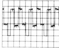
⑪ 4.5 Vp-p (H)
