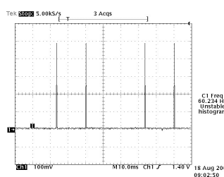
2 U201-#28 V-SYNC
