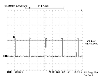
2 U201-#27 H-SYNC
