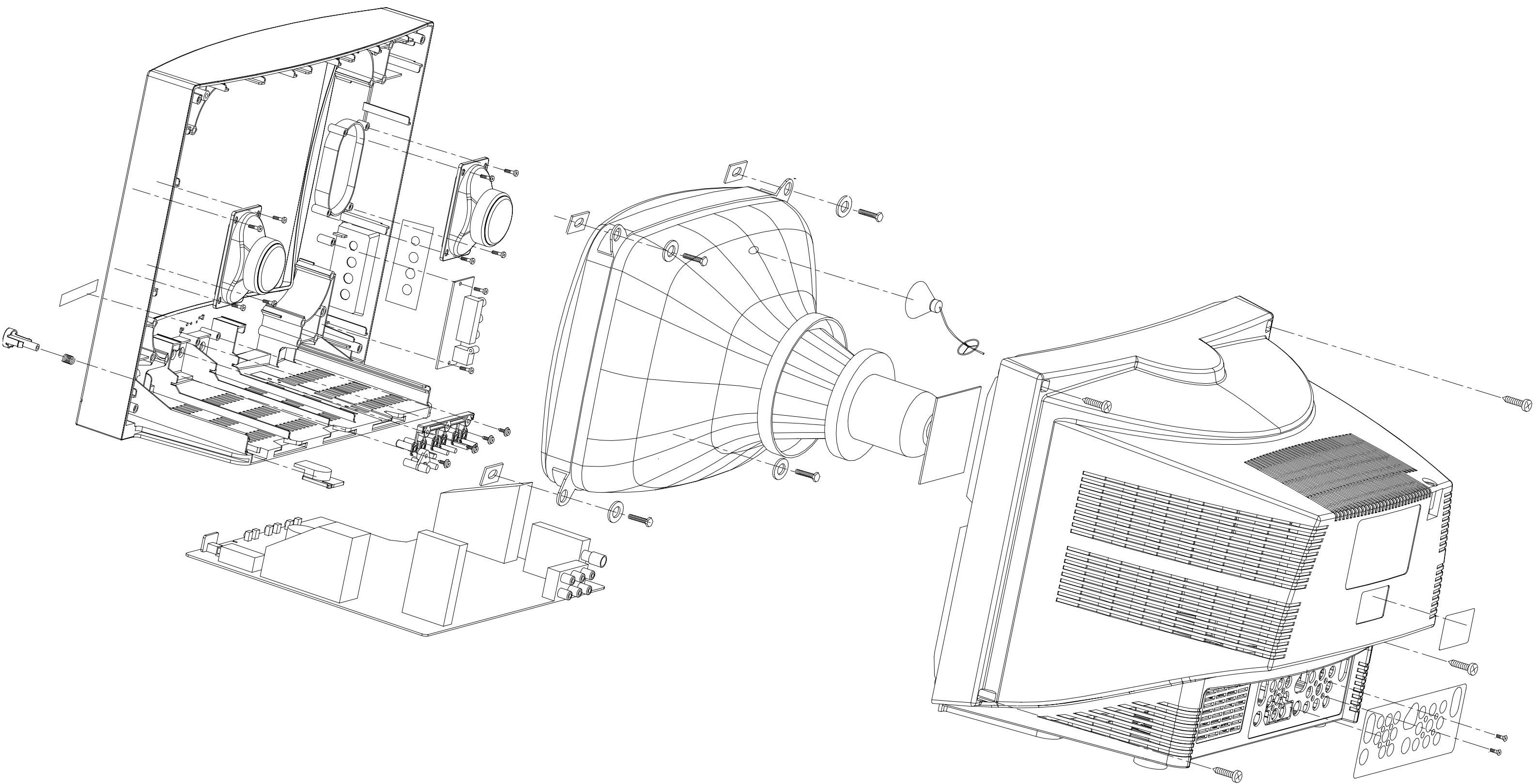
1427爆炸图
