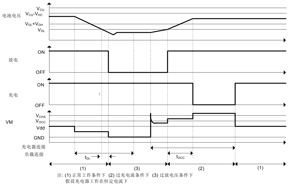
图 6. 过充电流检测
